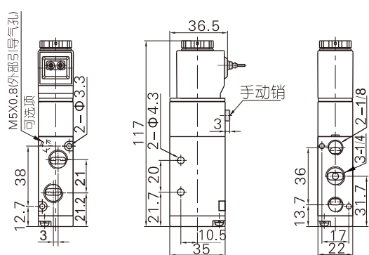
4V210出线式
