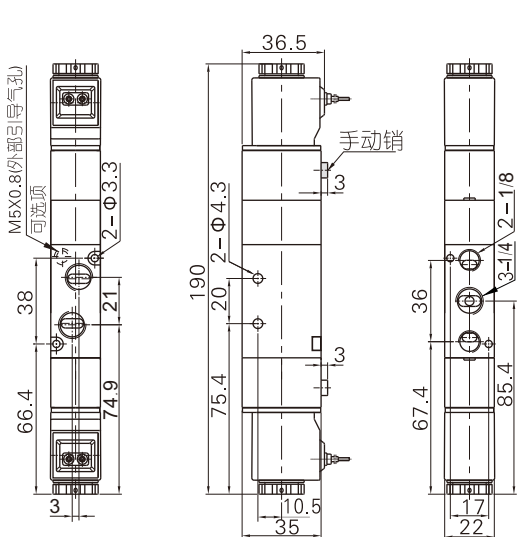
4V230出线式
