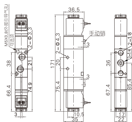
4V220出线式
