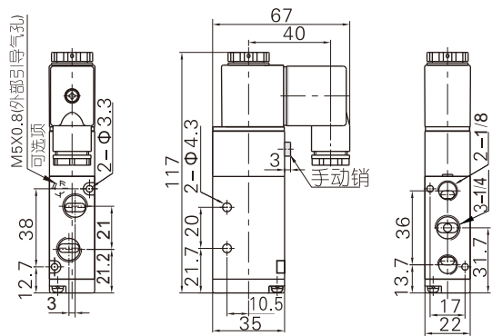
4V220DIN插座式
