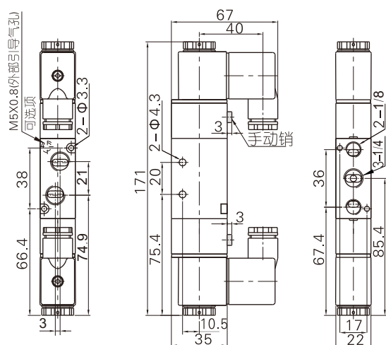
4V220DIN插座式
