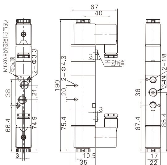
4V230DIN插座式
